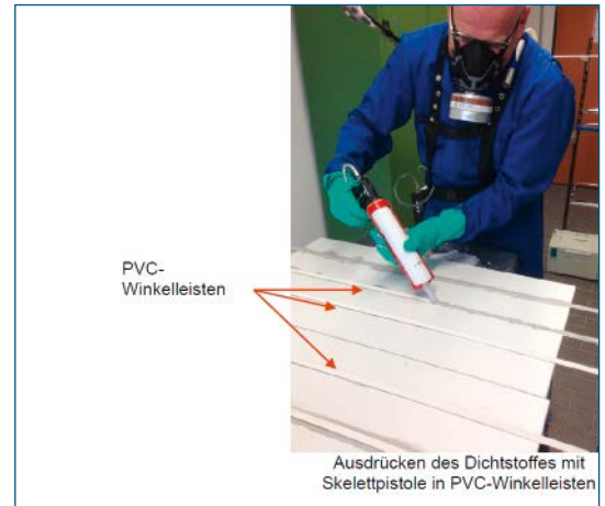
Abb. 1: Verarbeitung eines Dichtstoffes zu Beginn der Messung, Ausdrücken des Dichtstoffes mit Skelettpistole in PVC-Winkelleisten
