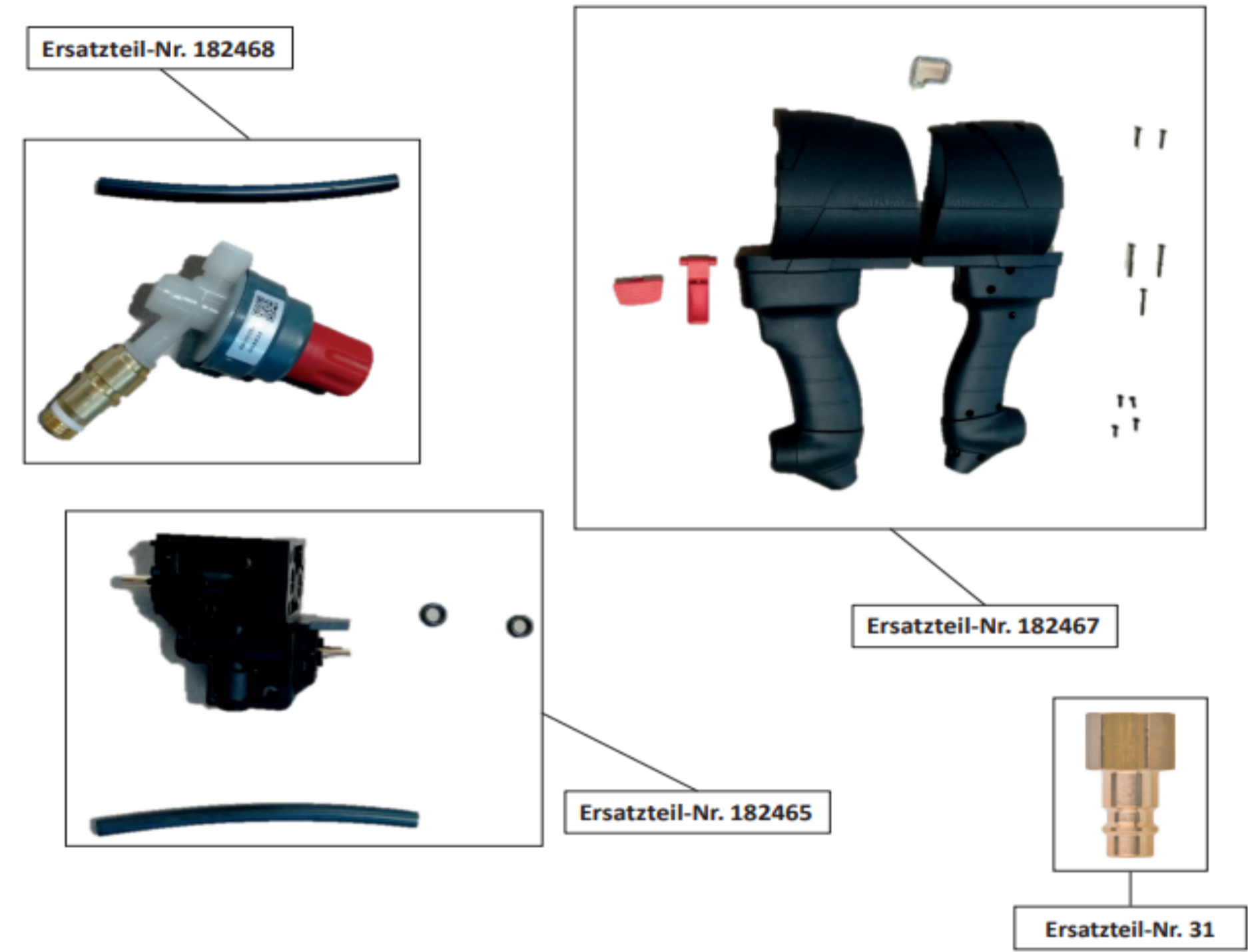
Ersatzteil Aufstellung für Pistole
