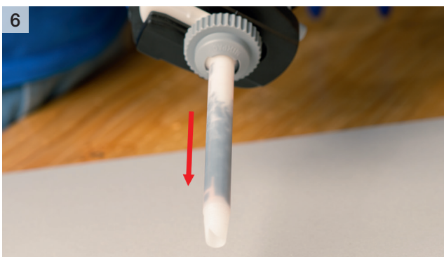
Befüllen des Statikmischers mit Klebstoff. Homogenität der Mischung prüfen (siehe verarbeitungsbegleitende Qualitätskontrollen 2K-Produkte)
