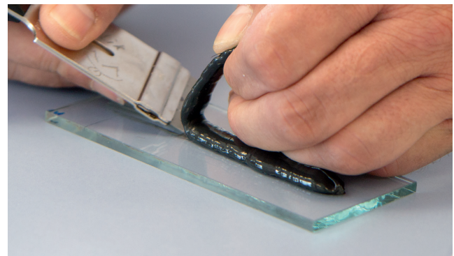
Einschneiden zwischen Klebstoff und Glasscheibe
