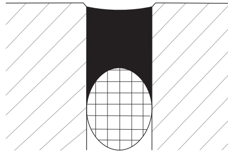
vorwiegend befahrene Fugen
