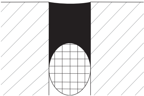
vorwiegend begangene Fugen
