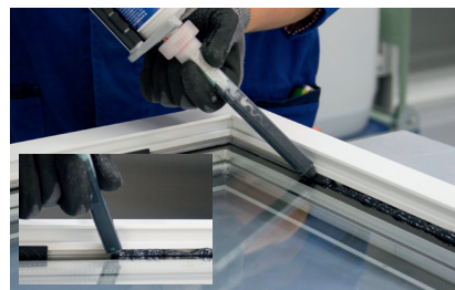
Befüllen des Falzgrundes mit Klebstoff
